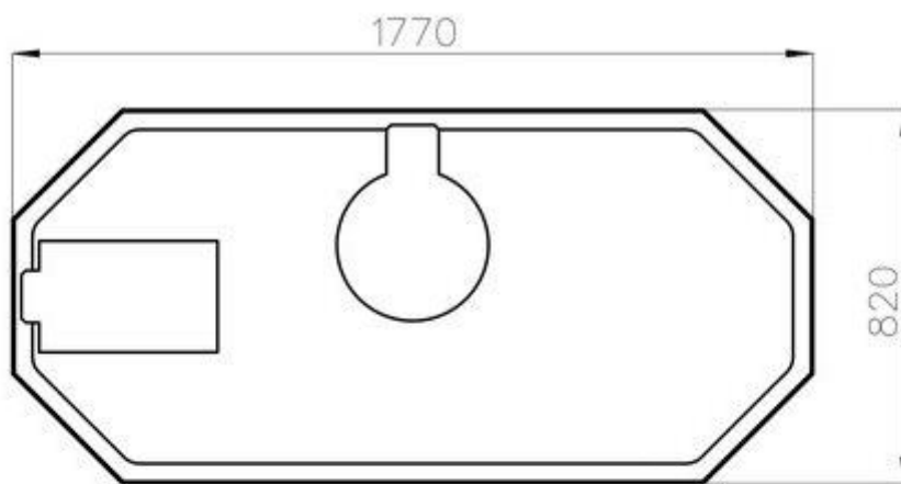
Draufsicht
